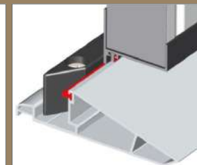
SEUIL BAS EN ALUMINIUM DRAINÉ
