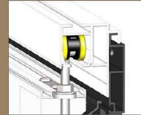
CHARIOT 4 ROULETTES SUR ROULEMENT AXE EN INOX
